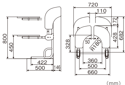
TST-100テーブルタイプ用の寸法
